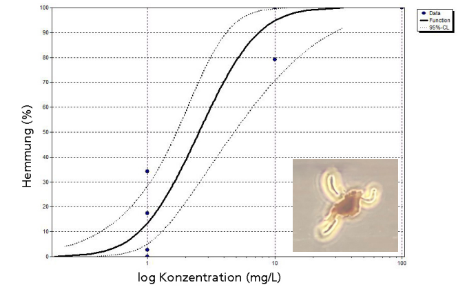
Abbildung 5: Mikroskopische Aufnahme der Interaktionen eines partikulären Polymers mit Algenzellen (OECD 201 Wachstumshemmtest mit Süßwasseralggen Raphidocelis subcapitata ) und die korrespondierende Dosiswirkungsbeziehung (Darstellung mit ToxRat®).
